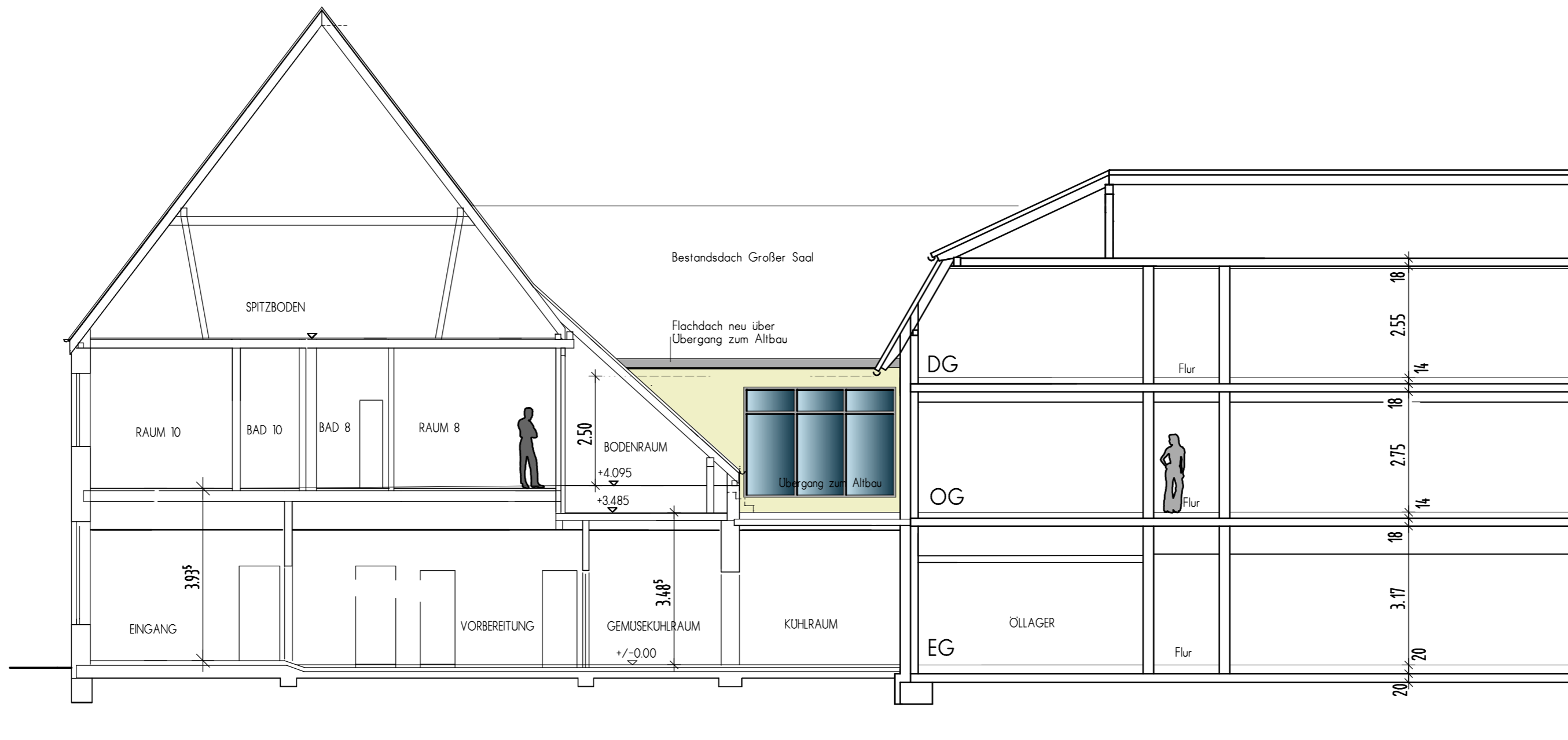
LÄNGSSCHNITT GEPLANT
